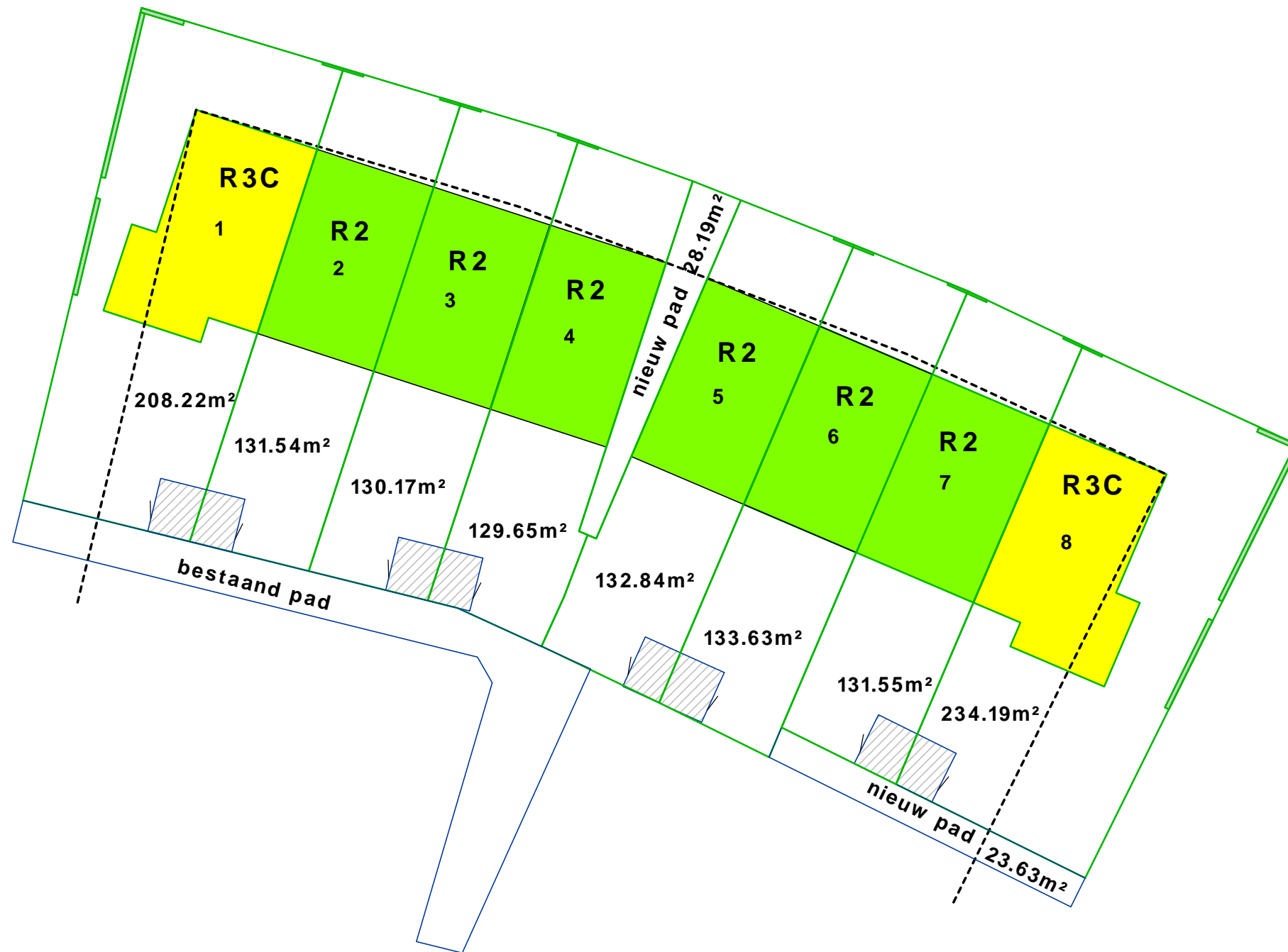
situatie 1:250
